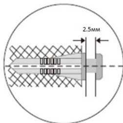
Рисунок 2.4 Установка шурупов
